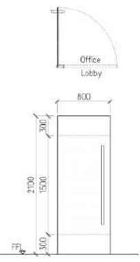
7 DOOR SCHEDULE SCALE: A-3 1:50 MTS
