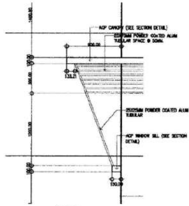
2 BLOW-UP SECTION SCALE: A-3 NTS
