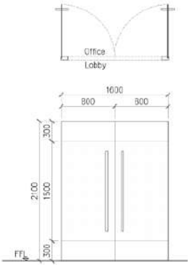
6 DOOR SCHEDULE SCALE: A-3 1:50 MTS
