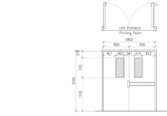
8 DOOR SCHEDULE SCALE: A-3 1:50 MTS
