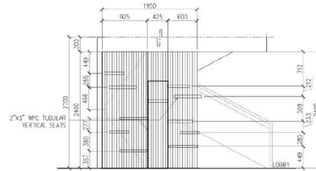
3 SIDE ELEVATION SCALE: 1:50 MTS
